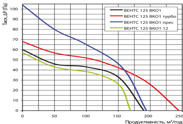
Рис. 6. Залежність продуктивності вентилятора
