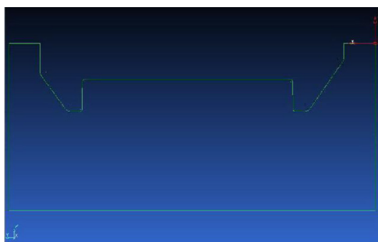
Рис. 18. Профіль матриці
