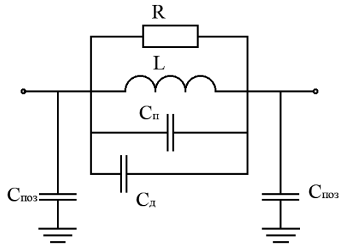
Рис. 4. Схема заміщення для визначення додаткової ємності
