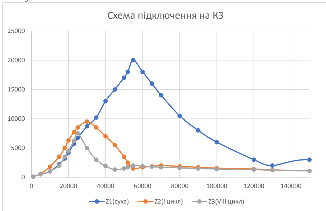
Рис. 3. Частотні характеристики двигуна зняті по схемі КЗ
