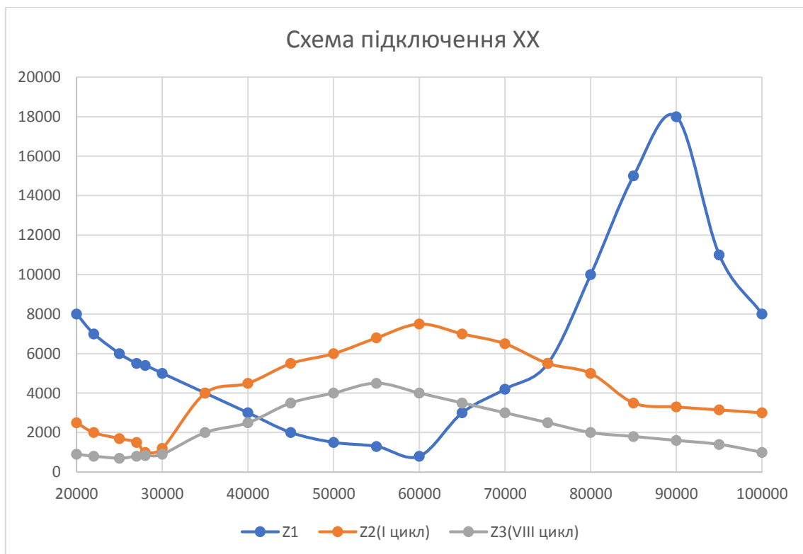
Рис. 2. Частотні характеристики двигуна зняті по схемі ХХ
